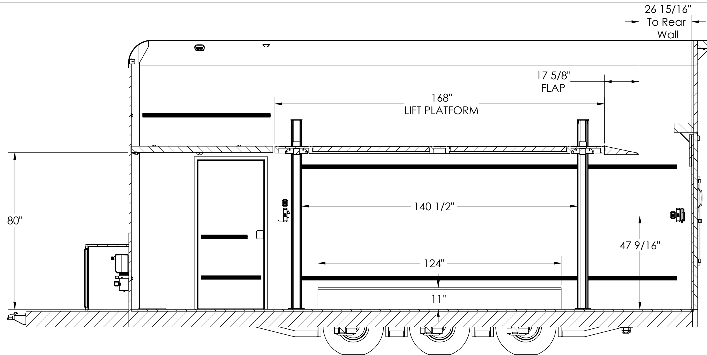
SECTION A-A
